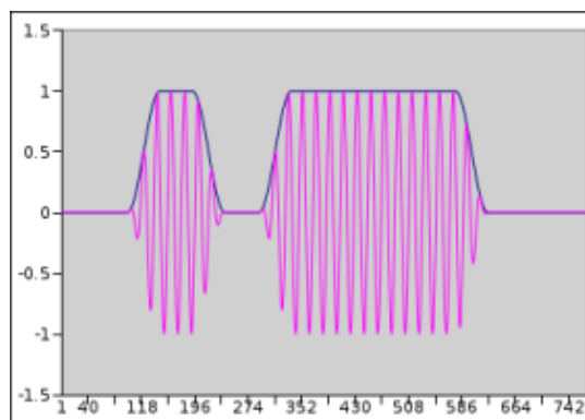
Figure 4.109 Dash/Dot = 3.0, Edge = 6 msec
