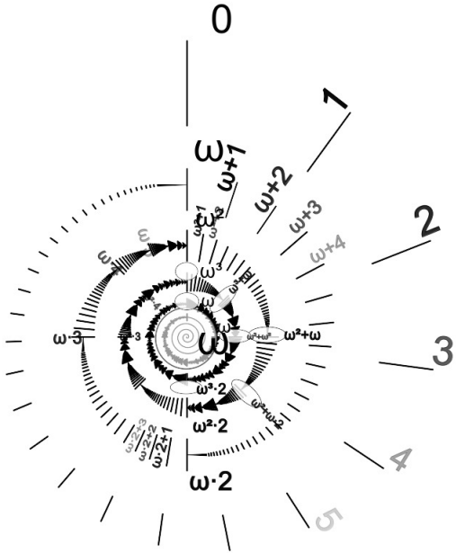
图 6.22: 无限伸展的无穷序数
