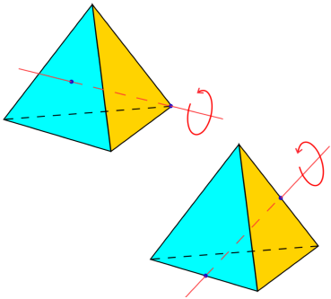
图 19: 正四面体的两种对称轴
