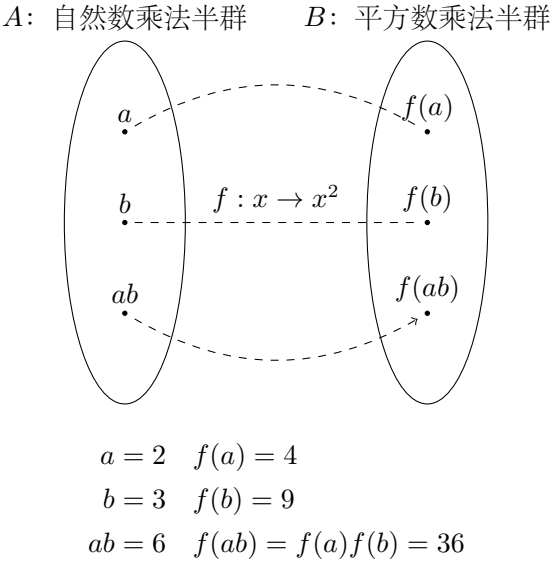
图 3.10: 同构
