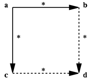
图 2.14: 丘奇-罗瑟定理的示意
