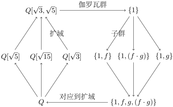
图 3.29: 伽罗瓦对应
