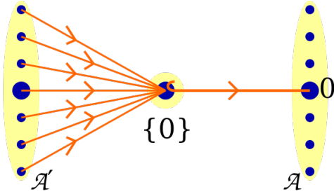
图 4.12: 零对象
