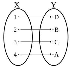
图 6.18: 集合间的一一对应
